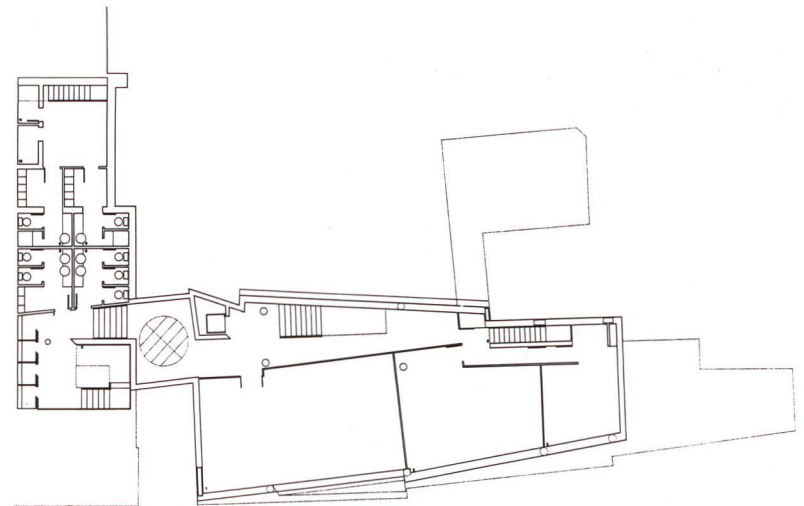
Planta sótano. Basement plan.
