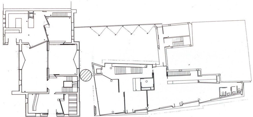
Planta baja. Ground plan.
